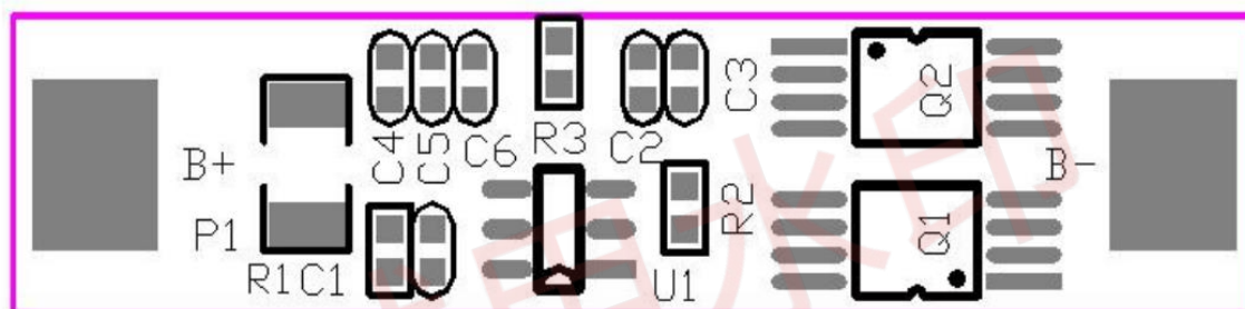
Bottom Layer
