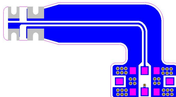
底层线路
