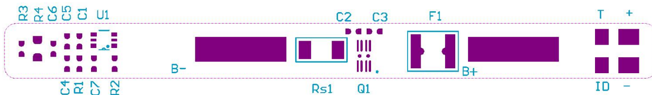
顶层线路
